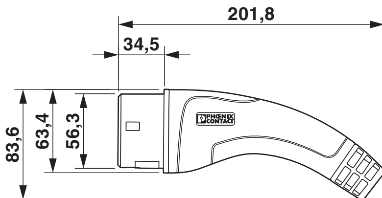
Dessin coté
