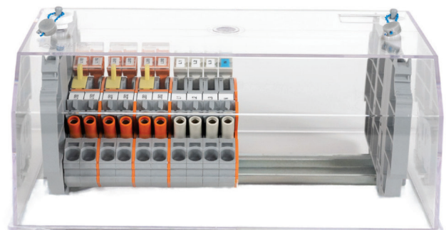
Modularität der Bestückung Klemmenblock: 2007-8875 2-Leiter-Trenn- und Messklemme: 2007-8811
