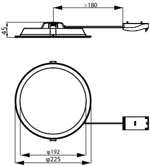
DN065B G4 LED20/830_840_865 19W D200 RD
