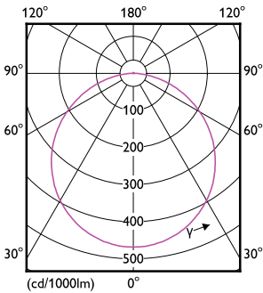
DN065B G4 LED20 CCT 19W D200 RD
