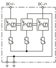
Prinzip Schaltbild DCU 2 YPV 1+2 1200 2M 1S MC4
