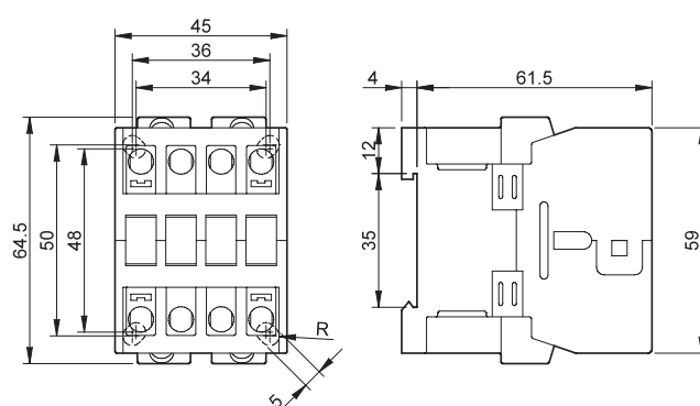
Tipo 6K.13-4350/4374 Morsetti a bussola
