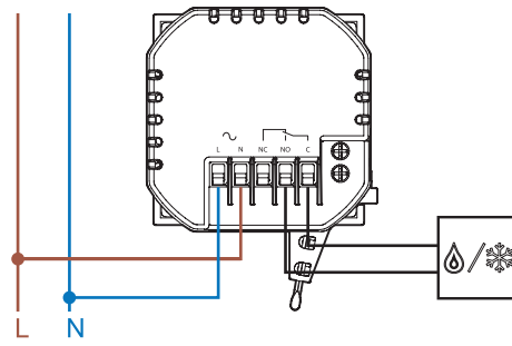
Anschlussbild standard
