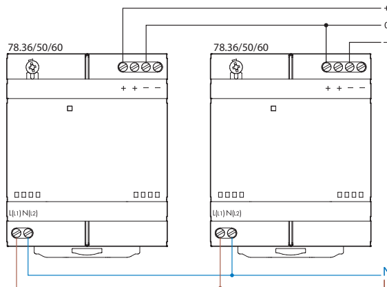
Collegamento a doppia polarità
