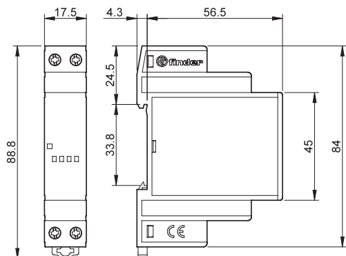
Tipo 78.25 Morsetti a bussola
