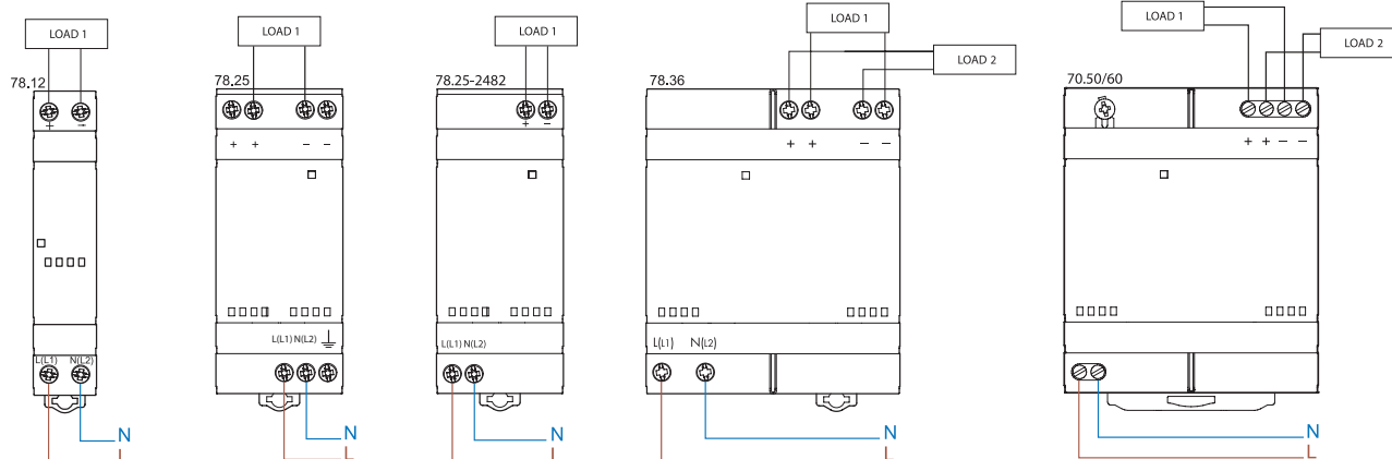
Collegamento a doppia polarità
