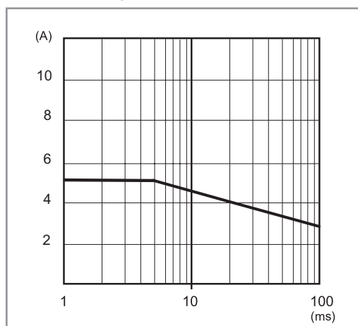
P78-4 Einschaltspitzenstrom-Belastbarkeit (78.60)
