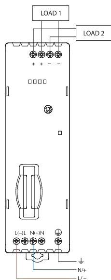
78.1B - Anschlussbild
