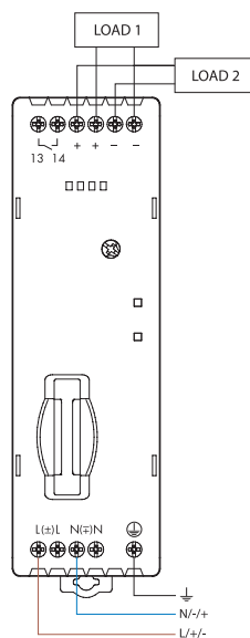
78.1D - Anschlussbild
