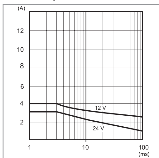
P78-2 Einschaltspitzenstrom-Belastbarkeit (78.25)
