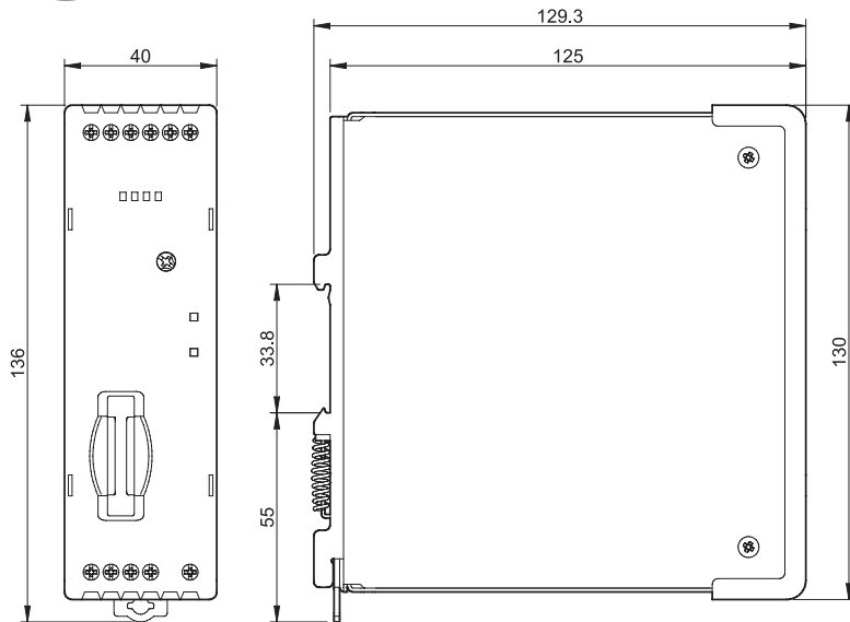
Typ 78.2E Käfigklemmen
