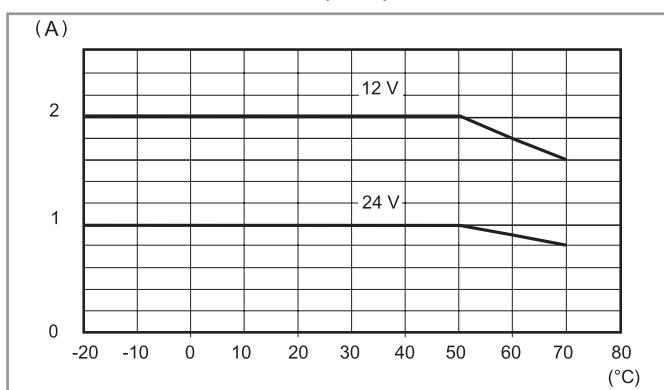
L78-2 Dauerstrom-Belastbarkeit (78.25)
