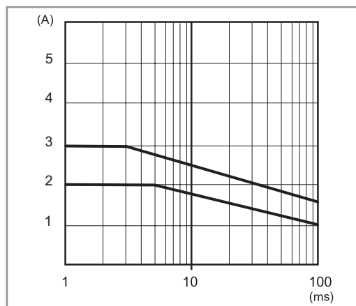
P78-2 Einschaltspitzenstrom-Belastbarkeit (78.25)
