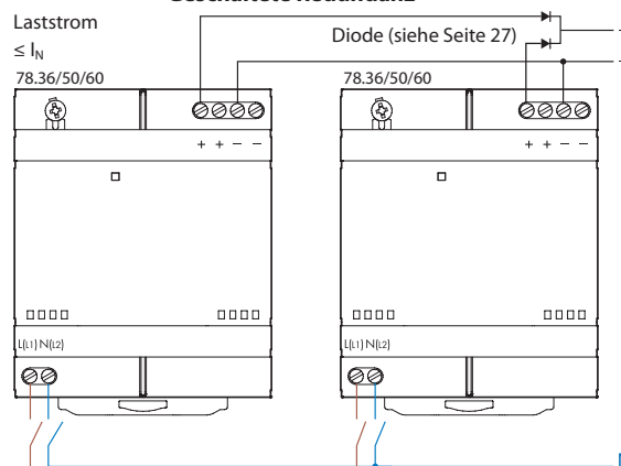
Geschaltete Redundanz
