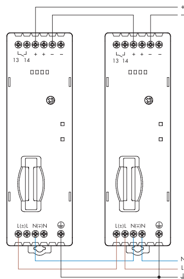
Serienschaltung zur Spannungsverdoppelung
