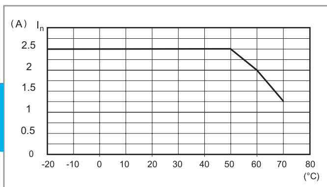
L78-4 Dauerstrom-Belastbarkeit (78.60)
