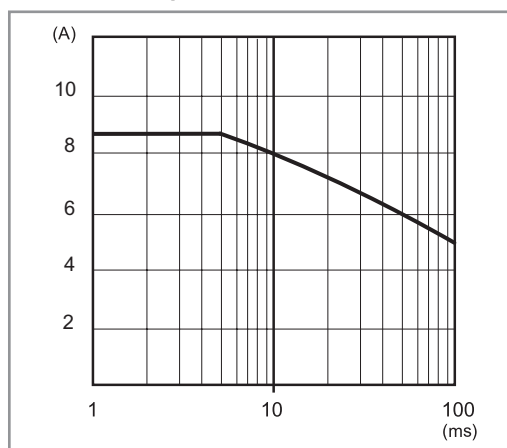
P78-5 Einschaltspitzenstrom-Belastbarkeit (78.50)
