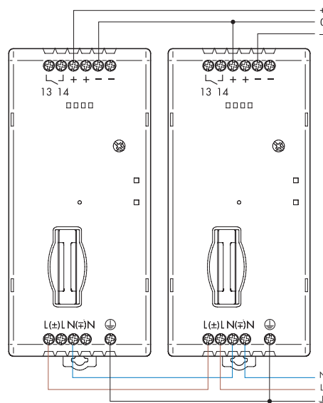
Serienschaltung zur Spannungsverdoppelung
