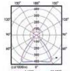
SP542P, BAP-tauglich
