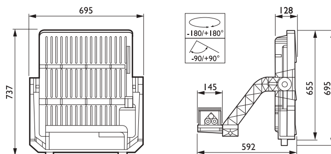
Ausführung BVP528. Abmessungen in mm
