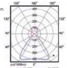
SP532P, BAP-tauglich
