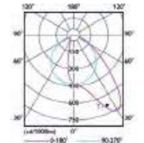
SP544P, asymmetrisch
