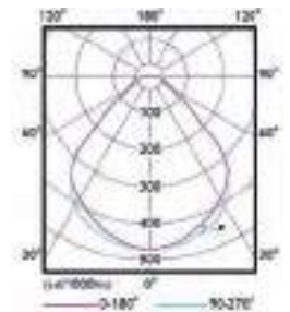
SM402C, quadratisch
