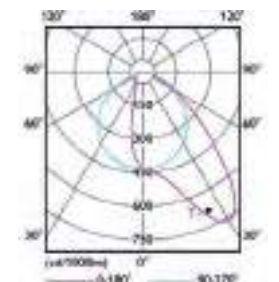
SP534P, asymmetrisch
