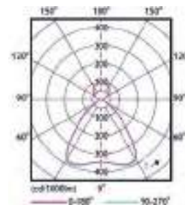
SP342P, PCS, adapté aux postes de travail équipés d'écrans
