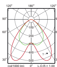
DA25W (Faisceau large double asymétrique, 25°)
