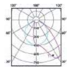
SP534P, asymétrique
