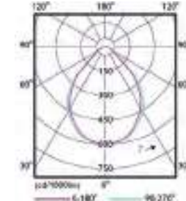
En option: SM340C, MLO, adapté aux postes de travail équipés d'écrans
