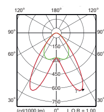
DA25N (Faisceau profond double asymétrique, 25°)
