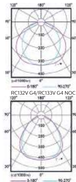
RC132V G4 / RC133V G4 OC, compatible avec les postes de travail équipés d'écrans
