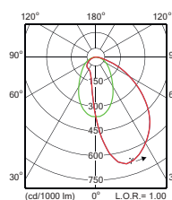
A20 (Faisceau asymétrique, 20°)
