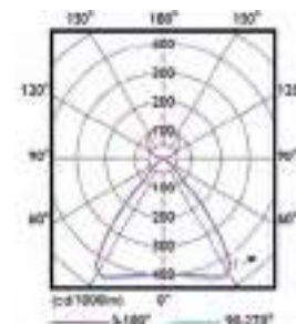
SP542P, adapté aux postes de travail équipés d'écrans
