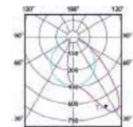
SP544P, asymétrique
