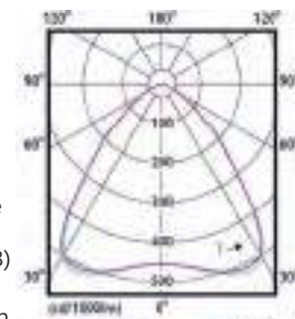
SM340C, PCS, adapté aux postes de travail équipés d'écrans
