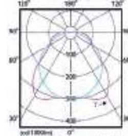
Dimmable WT120C G2
