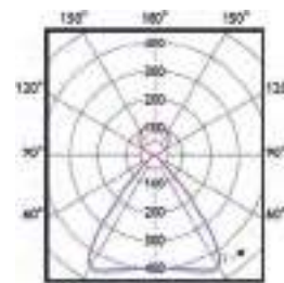
SP532P, adapté aux postes de travail équipés d'écrans
