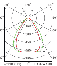
MB (Faisceau moyen)
