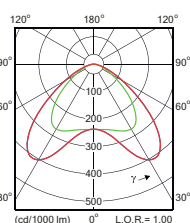
DA45 (Faisceau asymétrique double)
