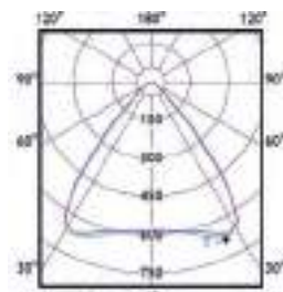
RC530B/RC532B, adapté aux postes de travail équipés d'écrans
