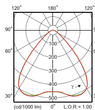
WB (Faisceau large)
