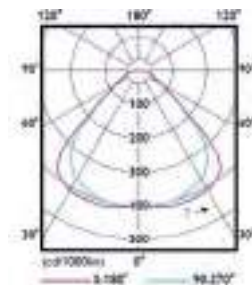
SM402C, long
