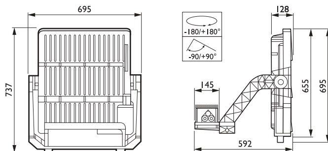
Modèle BVP528. Dimensions en mm
