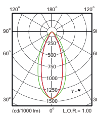
NB (Faisceau profond)
