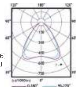
SM136V OC, adapté aux postes de travail équipés d'écrans
