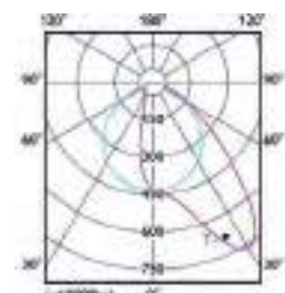
RC534B/RC535B, asymétrique
