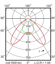
DA35W (Faisceau large double asymétrique, 35°)
