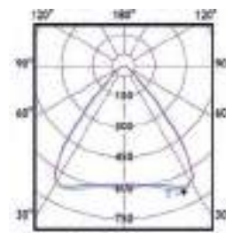
SM540C, adapté aux postes de travail équipés d'écrans
