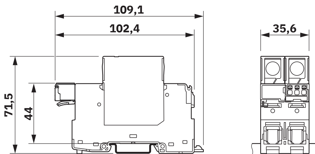
Disegno quotato
