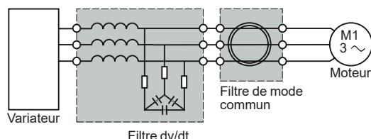
Variateur ATV340 avec filtre de mode commun
