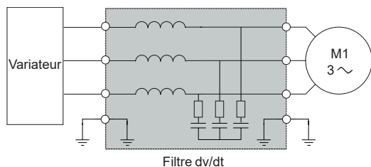
Variateur Altivar Machine avec filtre dv/dt
