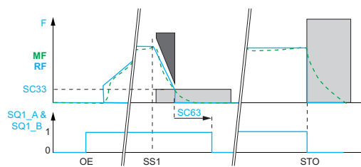
Activation de la fonction SBC
