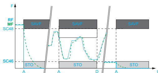
Activation de la fonction SLS
