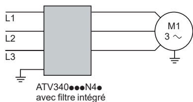
Variateur Altivar Machine ATV340 avec filtre CEM intégré
