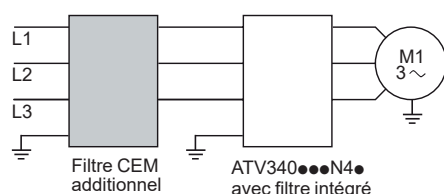
Variateur Altivar Machine ATV340 avec filtre CEM additionnel
