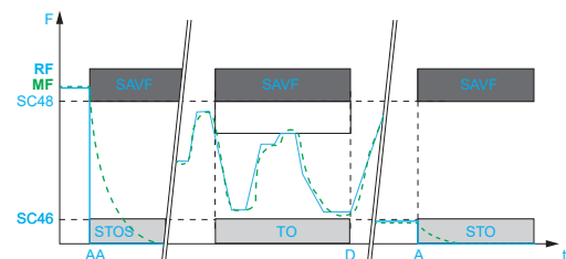
Activation de la fonction SLS
