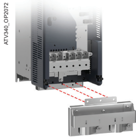
Type de montage en coffret VW3A47804 avec boîte de jonction amovible ATV340
