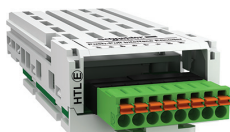
Module d'interface codeur HTL VW3A3424
