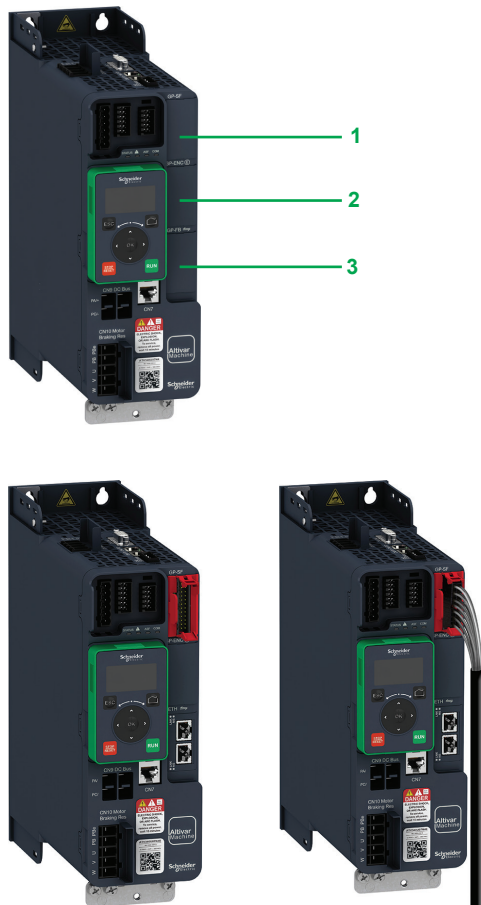
Module de sécurité à l'emplacement GP-SF
