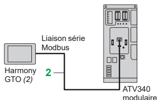
Exemple de raccordement d'un variateur modulaire ATV340 et d'un terminal de dialogue Harmony GTO via la liaison série Modbus
