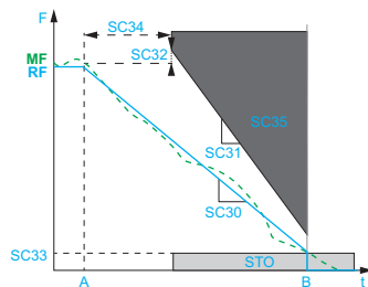
Activation de la fonction SS1
