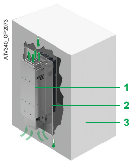
Kit de montage encastré NSYPTDS4 pour flux d'air séparé
