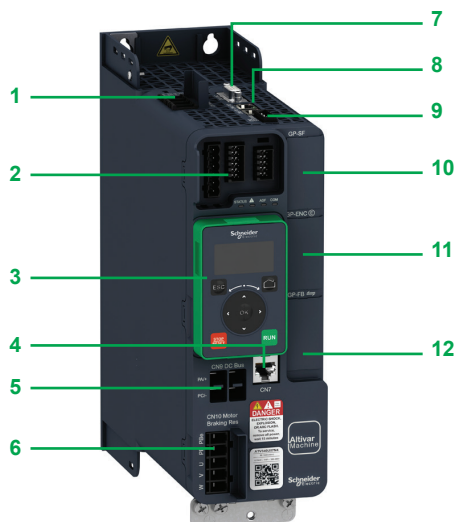
Variateur ATV340 Ethernet équipé du terminal graphique avec texte en clair
