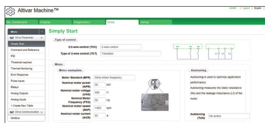
Onglet des paramètres du variateur
