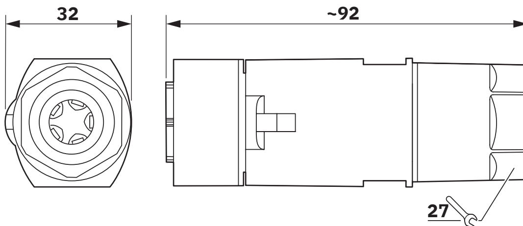
Disegno quotato
