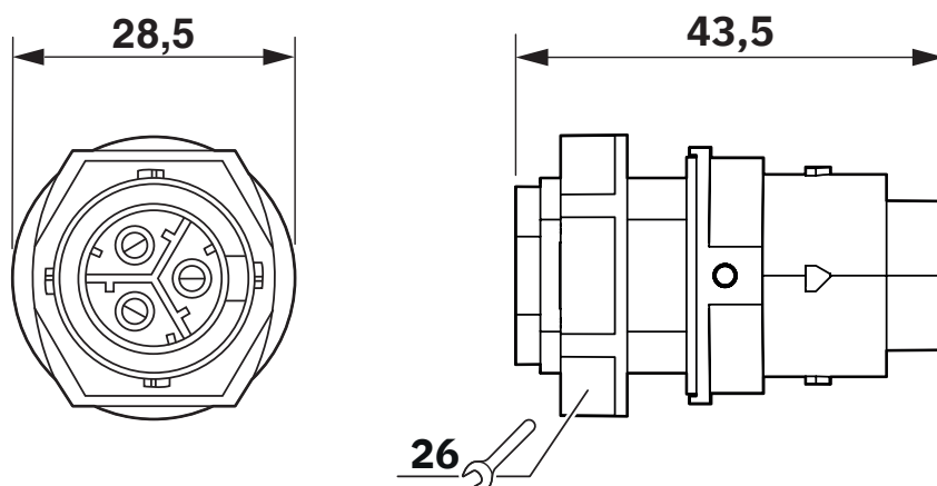
Disegno quotato
