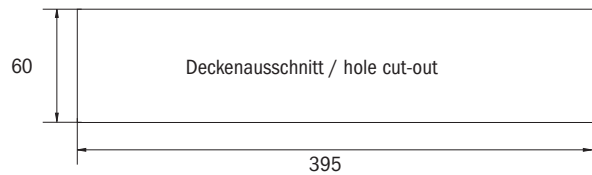
Découpe KXE cadre d'encastrement
