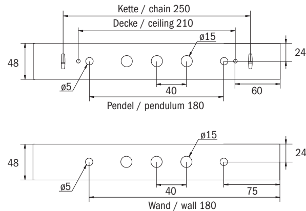
Dimensions KXE cadre d'encastrement
