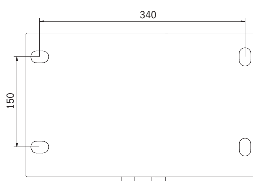
Distances de perçage AWV2-W
