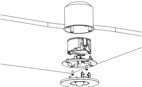
AWEE-xx-029 : prise pour commutateur nécessaire (non incluse dans la livraison)
