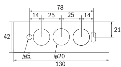
Distances de perçage AWKL plafond
