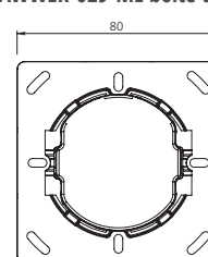
AWWER-029-ML boîte d'encastrement
