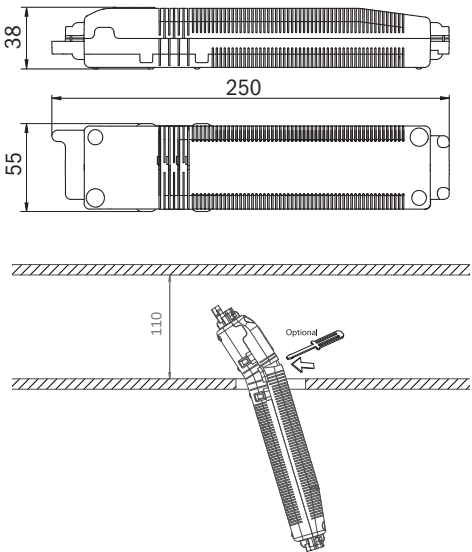
Boîtier électronique de batterie autonome (UH-1)
