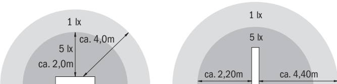
Répartition lumineuse KSC013 – mesurée à 1 m au-dessus du sol, hauteur de montage du luminaire 2,20 m
