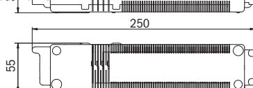
Boîtier électronique pour luminaires à batterie autonome
