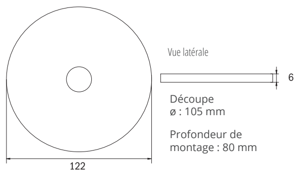
Dimensions et découpe AWIL-E (batterie autonome & batterie centralisée)
