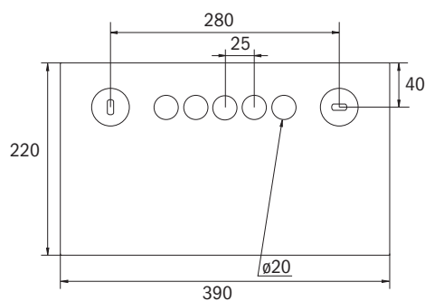
Distances de perçage AWKL mur
