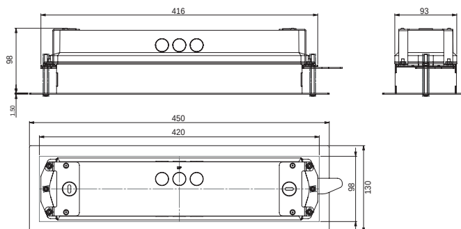
Distances de perçage AWKWI
