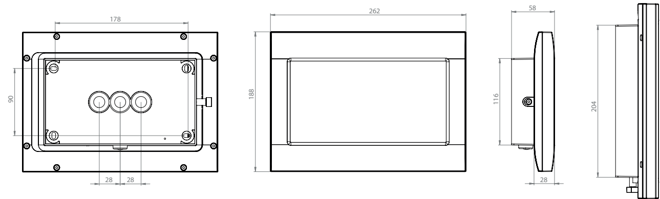
Dimensions et distances de perçage
