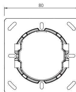
AWWEF-029(ML) boîte d'encastrement
