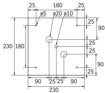
Distances der perçage AWWX
