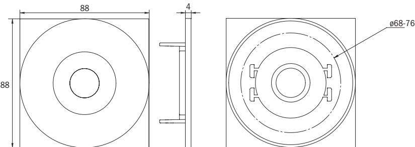
Découpe AWEE-R / AWEE-Q
