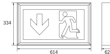
Dimensions AWLS mur
