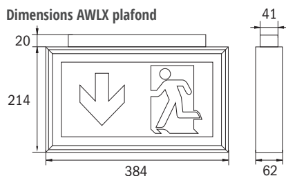
Dimensions AWLX plafond
