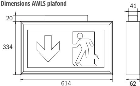
Dimensions AWLS plafond
