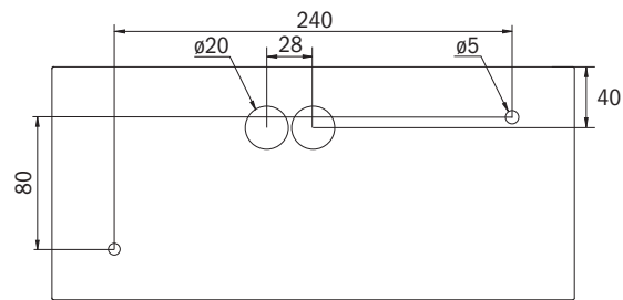
Distances de perçage AWZAW
