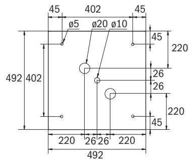
Distances der perçage AWWX
