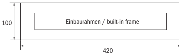
Dimensions KXE cadre d'encastrement
