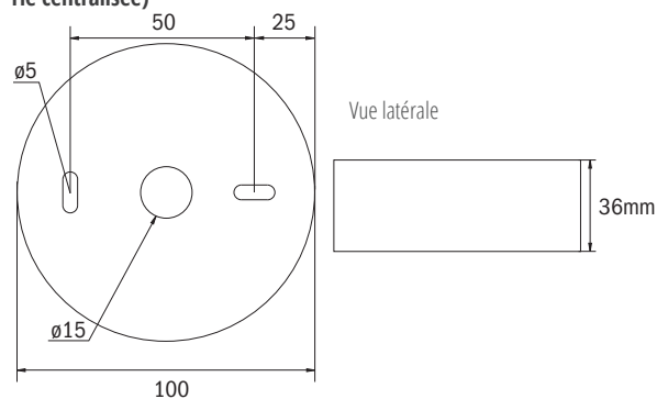
Dimensions & distances de perçage AWIL-D (batterie autonome & batterie centralisée)
