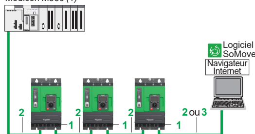
Démarreur progressif ATS480 + module VW3A3720
