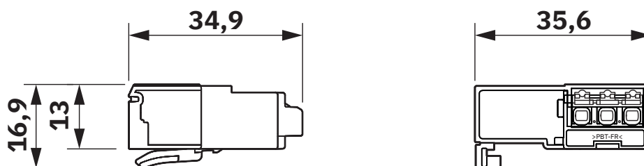
Disegno quotato
