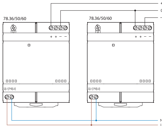
Serienschaltung zur Spannungsverdoppelung
