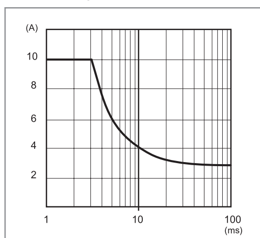
P78-4 Einschaltspitzenstrom-Belastbarkeit (78.60)
