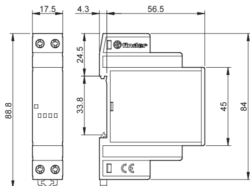
Typ 78.36 / 78.50 / 78.60 Schraubklemmen
