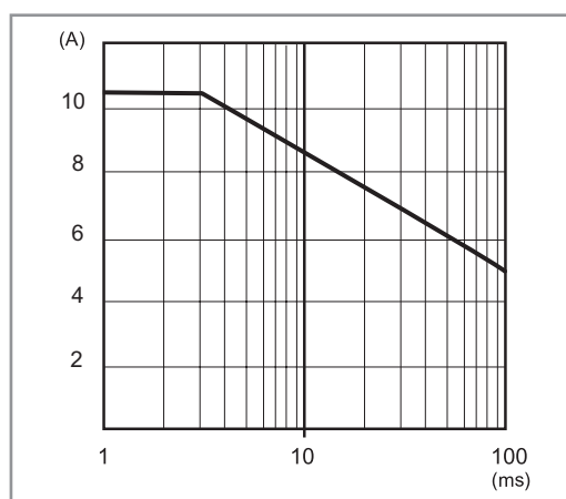
P78-5 Einschaltspitzenstrom-Belastbarkeit (78.50)
