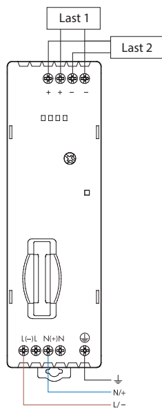
78.1B - Anschlussbild
