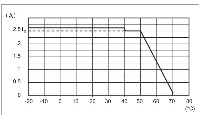
L78-4 Dauerstrom-Belastbarkeit (78.60)
