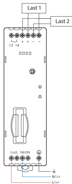
78.1D - Anschlussbild
