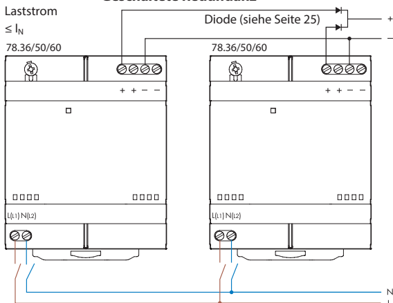
Geschaltete Redundanz
