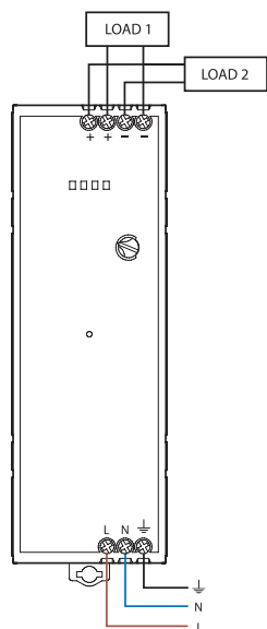
Schaltbild für 78.1A
