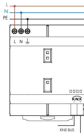
Schaltbild für 78.2K
