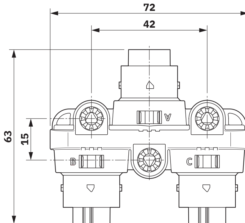
Dessin coté
