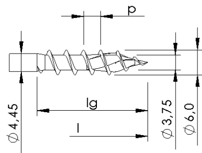
Ohne Gewindevariation, mit Spitzenrippen
