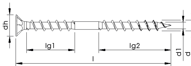
Unterkopfgewinde ohne Variation, ohne Schaftrippen, mit Spitzenverzahnung
