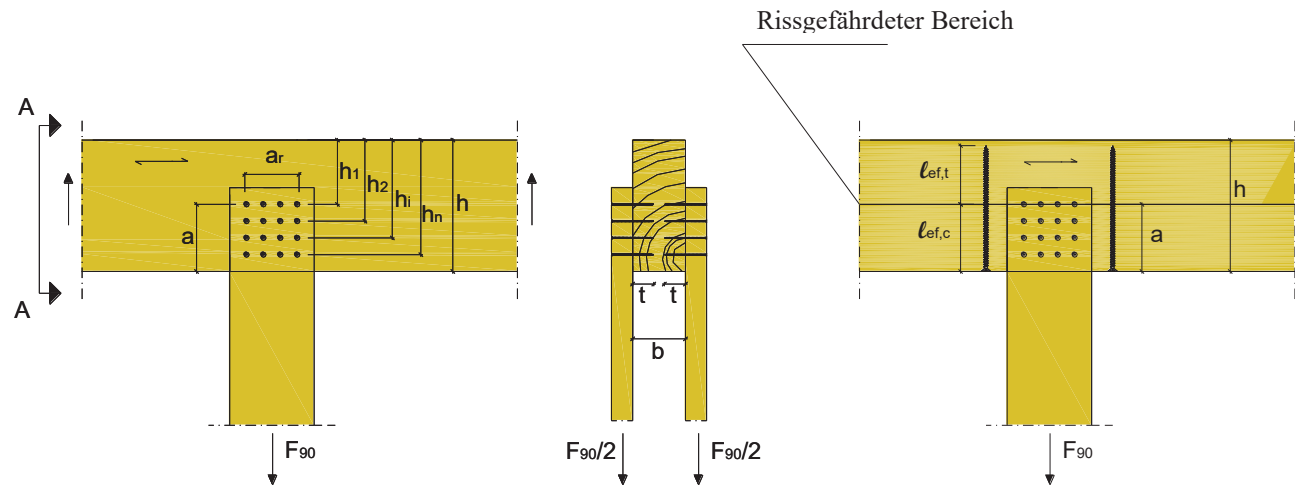
Abbildung 5: Beispiel für die Verstärkung eines Queranschlusses bei Beanspruchung rechtwinklig zur Faserrichtung
