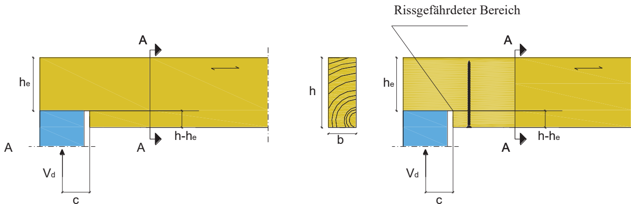
Abbildung 6: Beispiel für die Verstärkung eines ausgeklinkten Trägers bei Beanspruchung auf Zug
