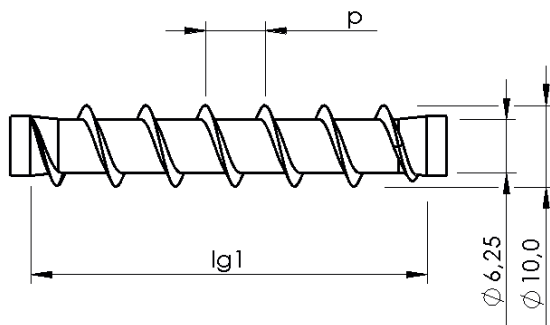
Unterkopfgewinde
