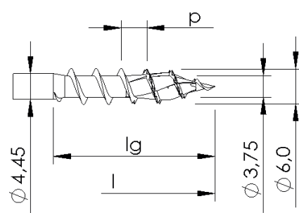
Ohne Gewindevariation, mit Spitzenverzahnung und -rippen
