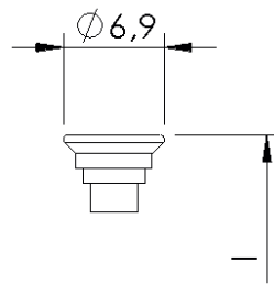
Stufenkopf
