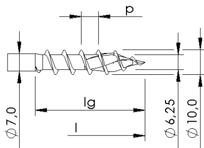
Mit und ohne Gewindevariation, mit Spitzenrippen
