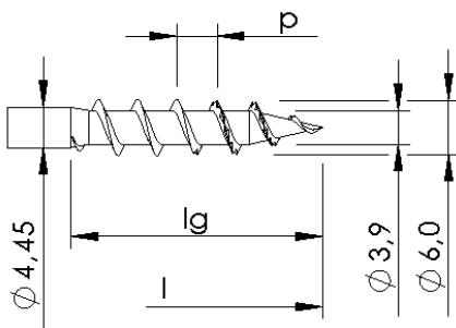
Mit und ohne Gewindevariation, mit Spitzenverzahnung
