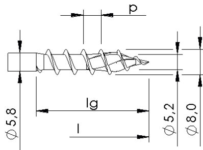
Mit und ohne Gewindevariation, mit Spitzenrippen
