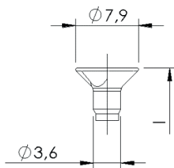
Flachsenkopf mit Kopfloch- bohrung, mit und ohne Frästaschen
