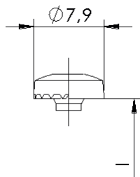
Panhead mit und ohne Unter- kopffräsrippen
