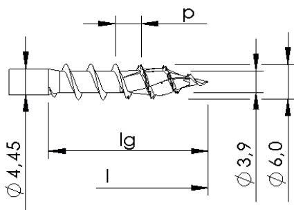
Mit und ohne Gewindevariation, mit Spitzenverzahnung und -rippen
