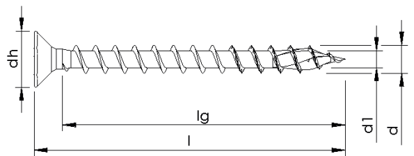
Vollgewinde ohne Variation, mit Spitzenrippen und -verzahnung
