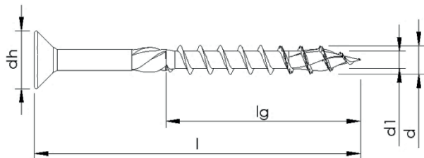
Teilgewinde ohne Variation, mit Schaftrippen, Spitzenverzahnung und Spitzenrippen
