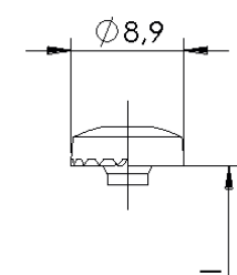
Panhead mit und ohne Unterkopffräsrip- pen
