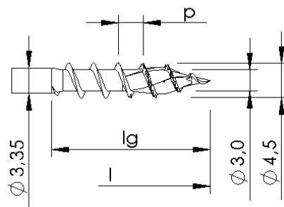
Mit und ohne Gewindevariation, mit Spitzenverzahnung und -rippen
