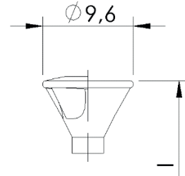
Flachsenkopf 60 / 75° mit und ohne Linse, mit und ohne Frästaschen
