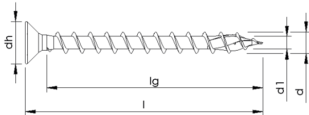
Vollgewinde ohne Variation, mit Spitzenrippen
