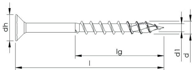
Teilgewinde ohne Variation, ohne Schaftrippen, mit Spitzenverzahnung und Spitzenrippen
