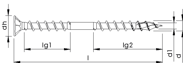
Unterkopfgewinde ohne Variation, ohne Schaftrippen, mit Spitzenverzahnung und Spitzenrippen
