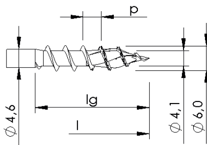
Ohne Gewindevariation, mit Spitzenverzahnung und -rippen
