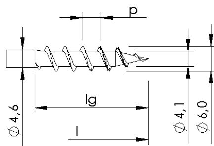
Ohne Gewindevariation, mit Spitzenverzahnung
