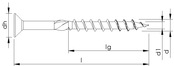
Teilgewinde ohne Variation, mit Schaftrippen und Spitzenverzahnung
