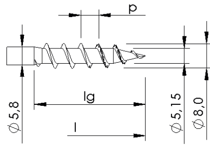
Mit und ohne Gewindevariation, mit Spitzenverzahnung
