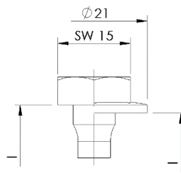
Sechskantkopf mit und ohne Scheibe
