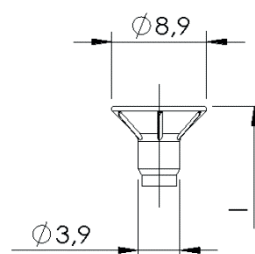
Flachsenkopf mit Kopfloch- bohrung, mit und ohne Fräsrip- pen
