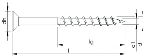
Teilgewinde ohne Variation, ohne Schaftrippen, mit Spitzenverzahnung
