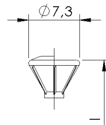
Flachsenkopf 60° / 75° mit und ohne Linse, mit und ohne Fräsrippen
