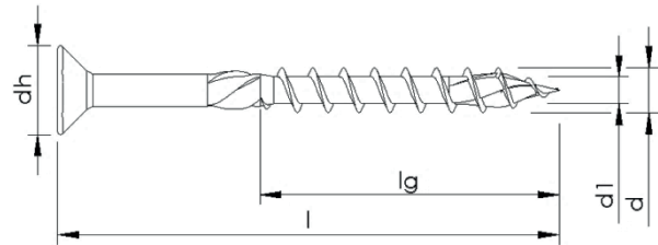
Teilgewinde ohne Variation, mit Schaftrippen und Spitzenrippen
