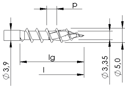
Mit und ohne Gewindevariation, mit Spitzenrippen
