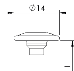
Linsentellerkopf mit aufgedicktem Schaft
