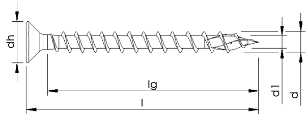
Vollgewinde mit Variation, mit Spitzenrippen
