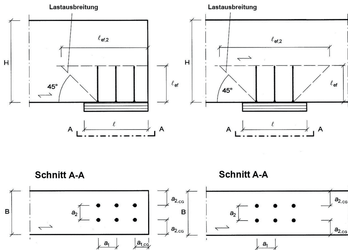
Abbildung 4: Verstärktes Endauflager (links) und verstärktes Zwischenauflager (rechts)
