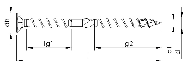
Unterkopfgewinde ohne Variation, mit Schaft-rippen, Spitzenverzahnung und Spitzenrippen
