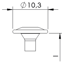
Rückwandkopf
