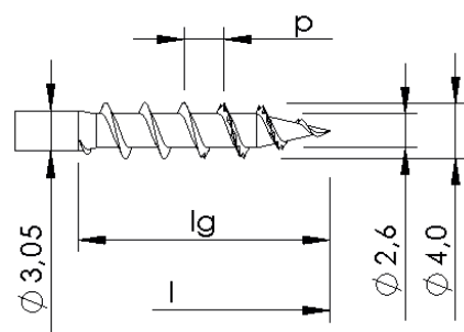
Mit und ohne Gewindevariation, mit Spitzenverzahnung
