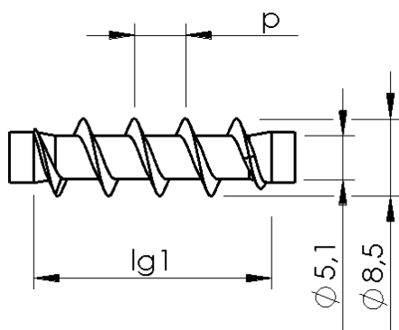
Unterkopfgewinde
