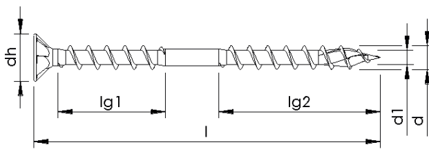
Unterkopfgewinde ohne Variation, ohne Schaftrippen, mit Spitzenrippen
