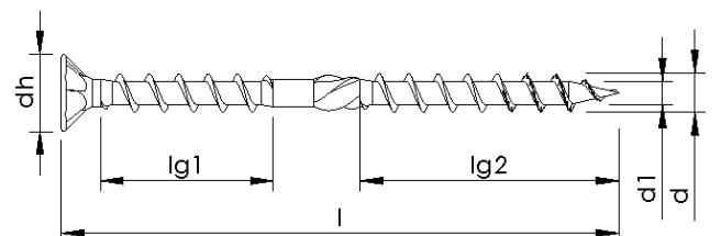
Unterkopfgewinde ohne Variation, mit Schaft-rippen und Spitzenverzahnung
