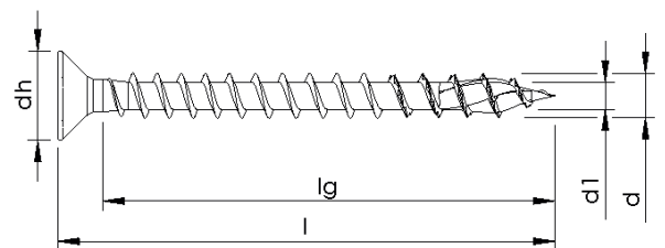
Vollgewinde mit Variation, mit Spitzenrippen und -verzahnung
