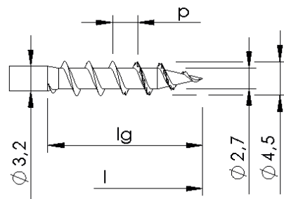
Mit und ohne Gewindevariation, mit Spitzenverzahnung
