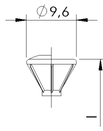
Flachsenkopf 60° / 75° mit und ohne Linse, mit und ohne Fräsrippen
