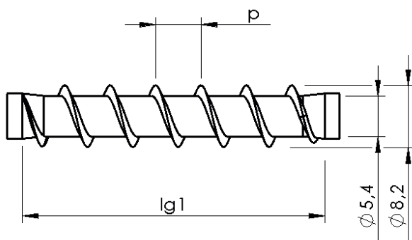
Unterkopfgewinde
