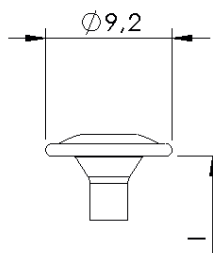
Rückwandkopf
