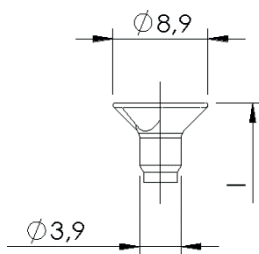
Flachsenkopf mit Kopfloch- bohrung, mit und ohne Frästaschen
