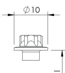
Außensechsrundkopf mit und ohne Scheibe
