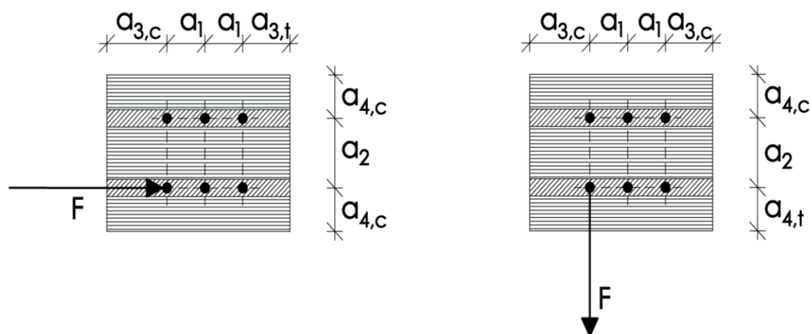
Abbildung 2: Definition der Achs-, End- und Randabstände der Schrauben in der Stirnfläche
