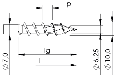
Mit und ohne Gewindevariation, mit Spitzenverzahnung und -rippen
