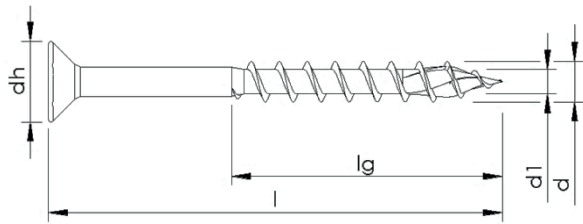
Teilgewinde ohne Variation, ohne Schaftrippen, mit Spitzenrippen
