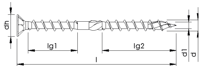
Unterkopfgewinde ohne Variation, mit Schaft-rippen und Spitzenrippen
