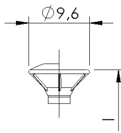
Flachsenkopf mit und ohne Linse, mit und ohne Fräsrippen
