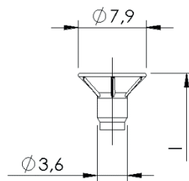
Flachsenkopf mit Kopfloch- bohrung, mit und ohne Fräsrip- pen
