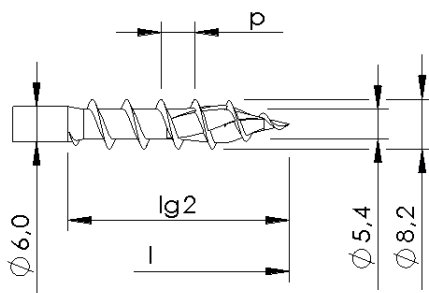
Ohne Gewindevariation, mit Spitzenrippen
