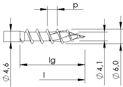
Ohne Gewindevariation, mit Spitzenrippen
