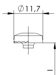
Panhead mit und ohne Unter- kopffräsrippen
