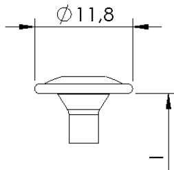
Rückwandkopf
