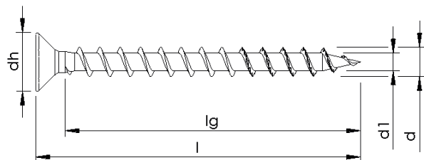
Vollgewinde ohne Variation, mit Spitzenverzahnung
