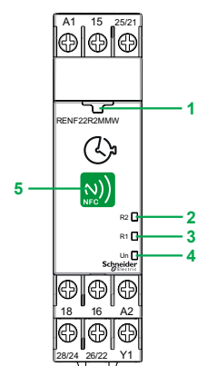
Relais temporisé NFC
