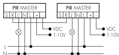
Funzionamento Master-Master
