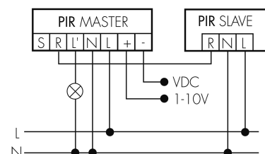
Funzionamento Master-Slave
