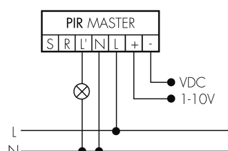
Funzionamento normale
