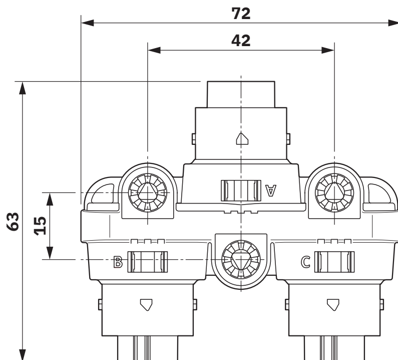
Disegno quotato
