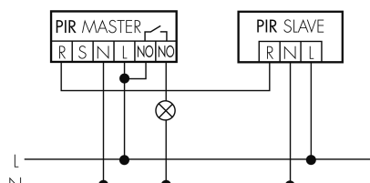
Fonctionnement Master-Slave
