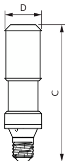
MAS LED SON-T EM 10.8Klm 65W 727 E40
