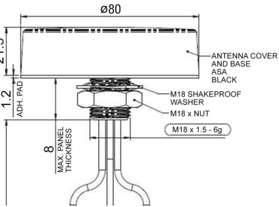
fig. 1. Abmessungen (mm)
