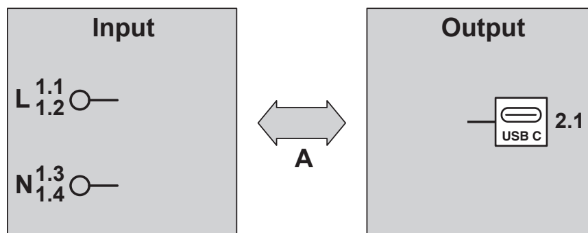
Disegno schema
