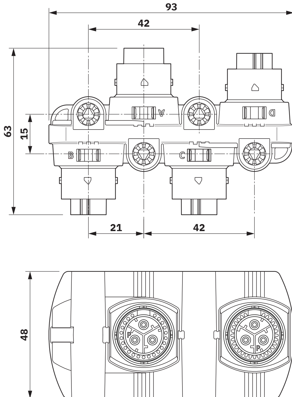
Disegno quotato
