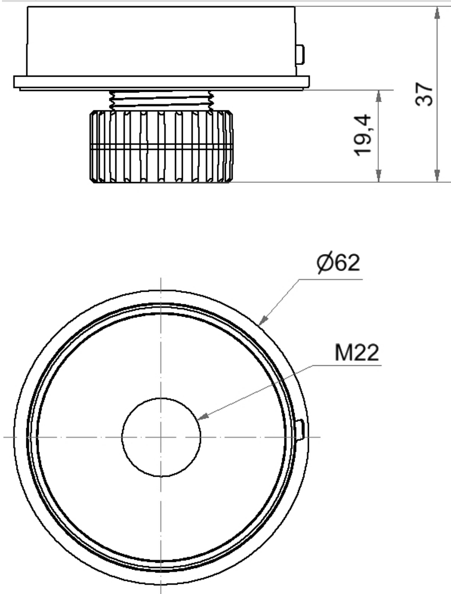
DIBUJO
