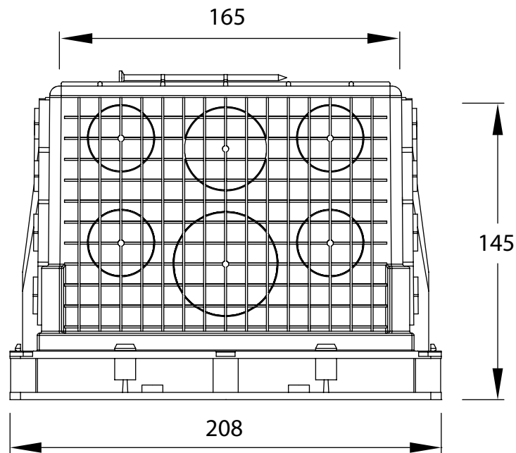
Abbildung: Multibox mit einem Aufsatzrahmen (E-No: 155011105)
