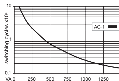
fig. 3. Gleichstrom-Grenzlastkurve
