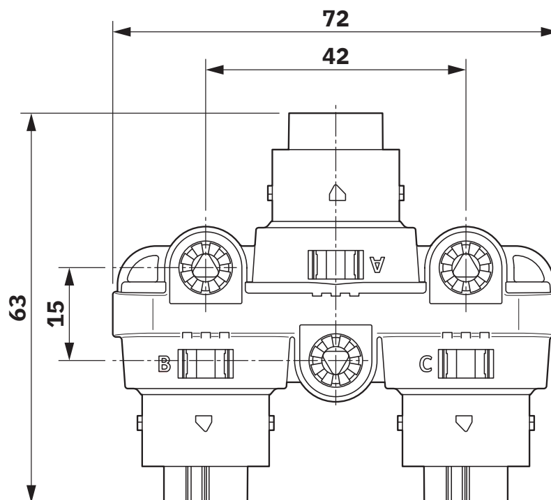
Dessin coté
