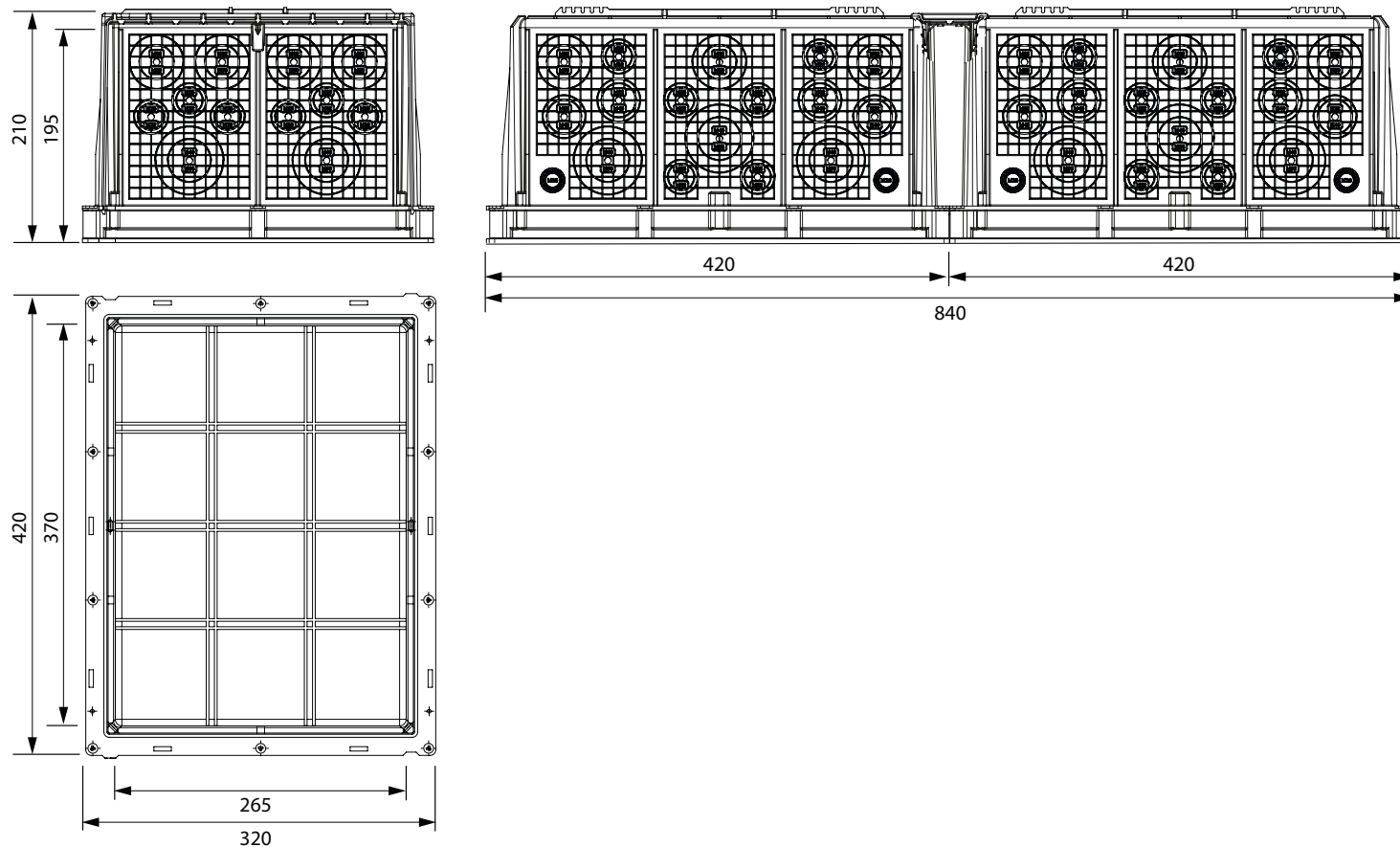
Abbildung: 2 Multibox XXL (520110) mit Verbinder (520300)
