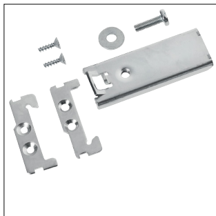
Befestigungsset SILAS für Hutschienen, Größe 00-1 für zwei Hutschienen
