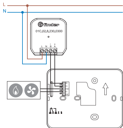
Anschlussbild
