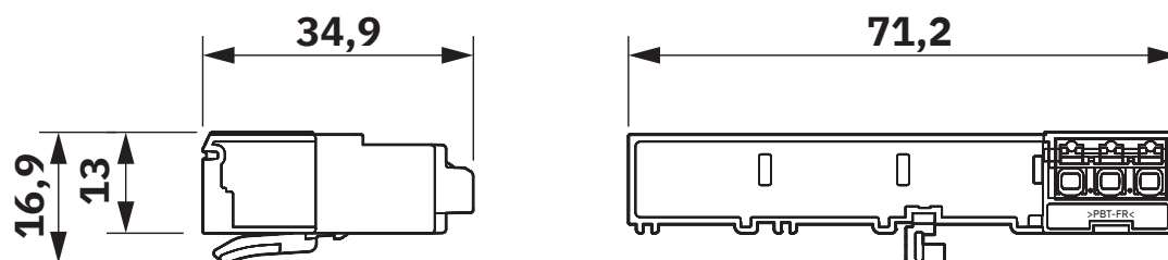
Disegno quotato
