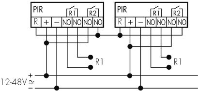
Funzionamento Master-Master
