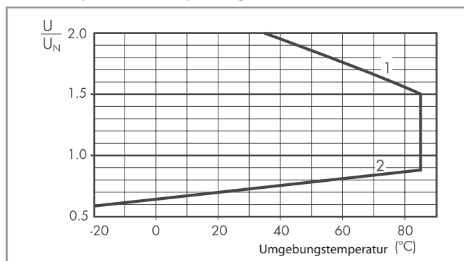
R 34 - DC Spulen-Betriebsspannungsbereich
