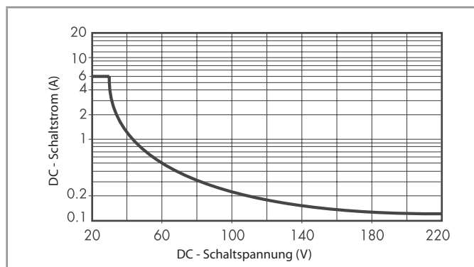
H 34 - Gleichstromschaltvermögen bei DC1 - Belastung
