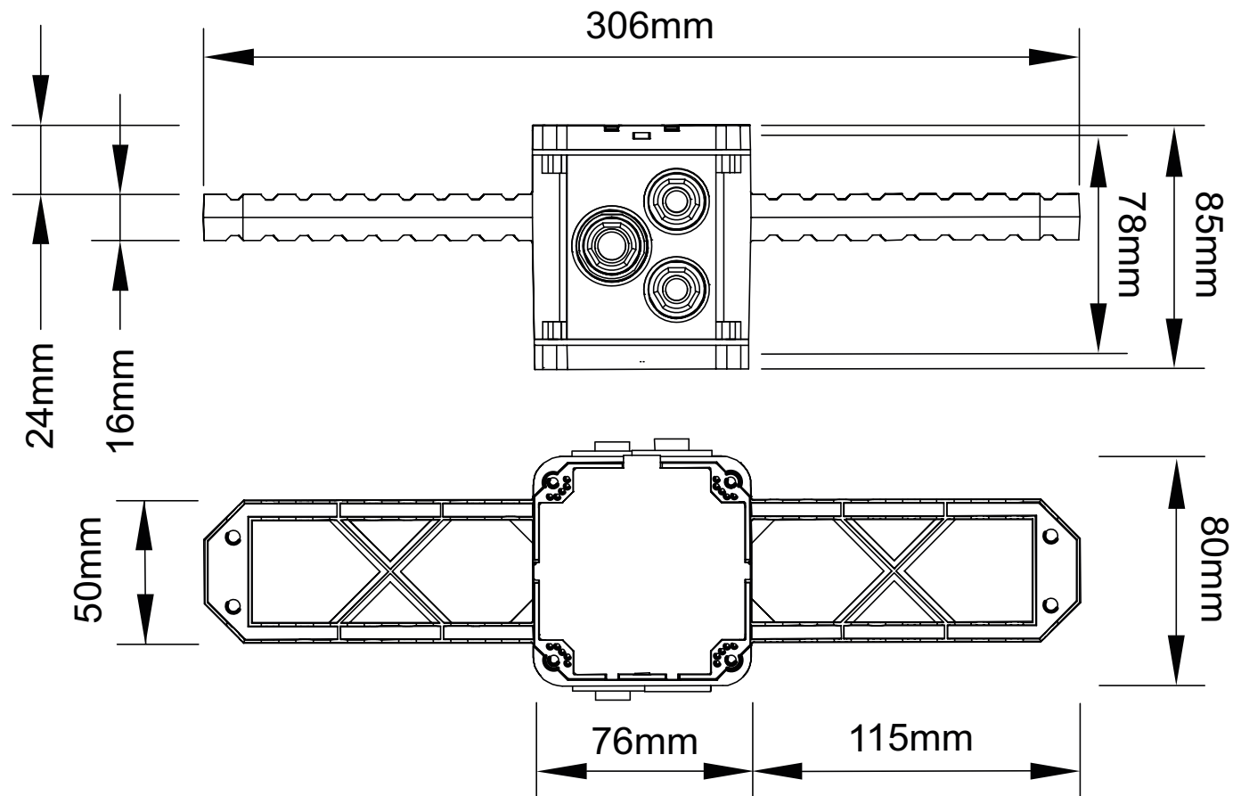
Abbildung: UP1 Flügeldose (E-No 372 702 939)
