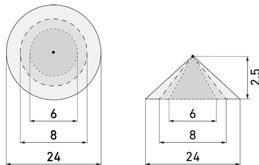
Dimensioni in m
