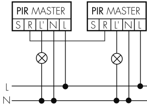
Normalbetrieb mit externem Taster
