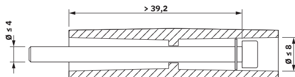
Maßzeichnung
