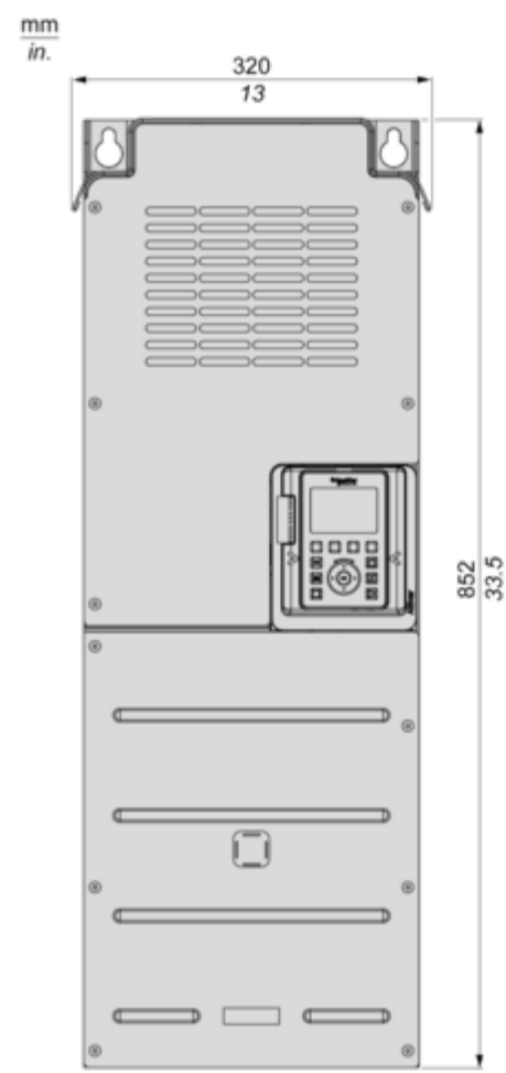
IP21-Umrichter ohne obere Abdeckung Rechtsseitige Ansicht und Vorderansicht
