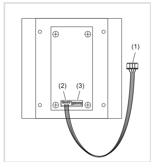
Figura 1: Vista posteriore
