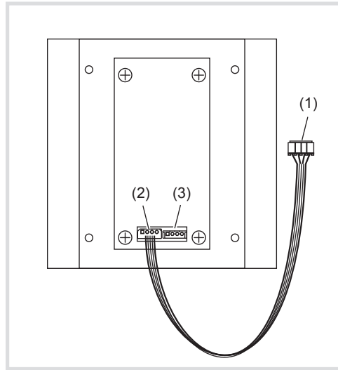
Afb. 1: achteraanzicht
