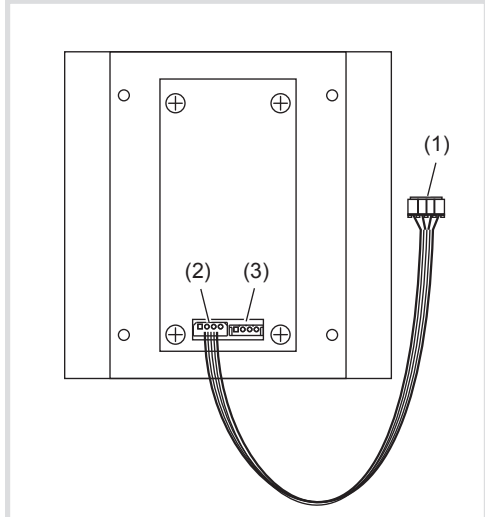
Bild 1: Rückansicht
