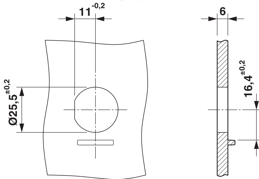
Disegno quotato
