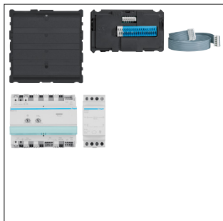
Kit électronique 2-fils AUDIO pour boites a lettres de 3eme fabricant
