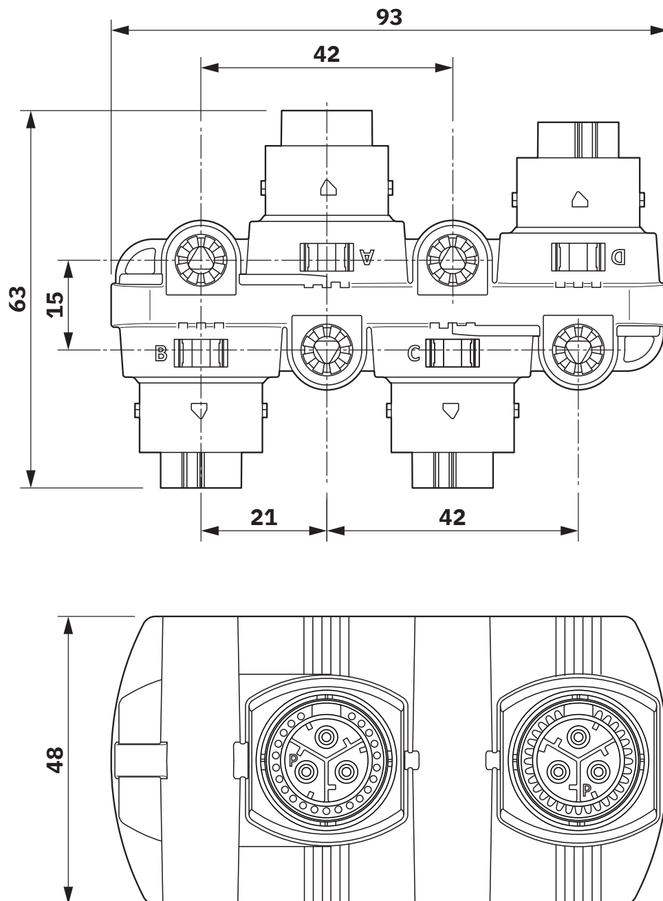
Disegno quotato
