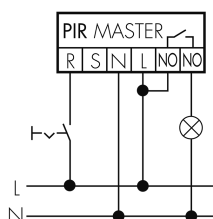
Funzionamento Master-Slave
