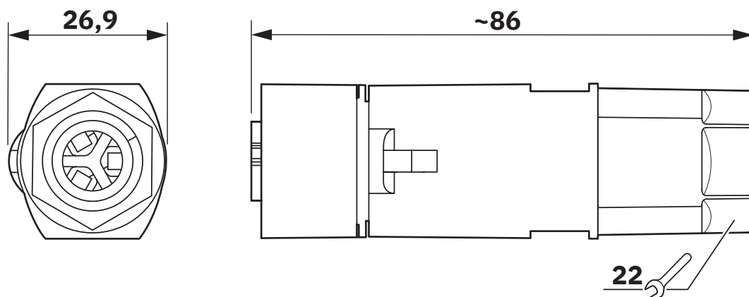
Disegno quotato
