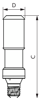
MAS LED SON-T EM 8.1Klm 50W 727 E40
